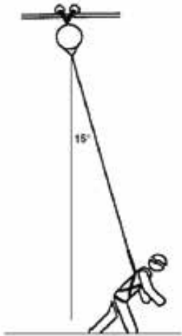
DAR2,5 ▶ arrotolatore a nastro con dissipatore di energia lunghezza da 0/250 cm
